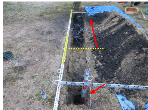
根は改良土内のみで伸長
