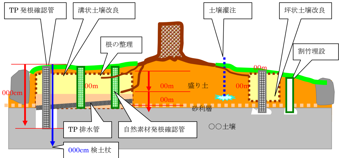
施工断面イメージ図
