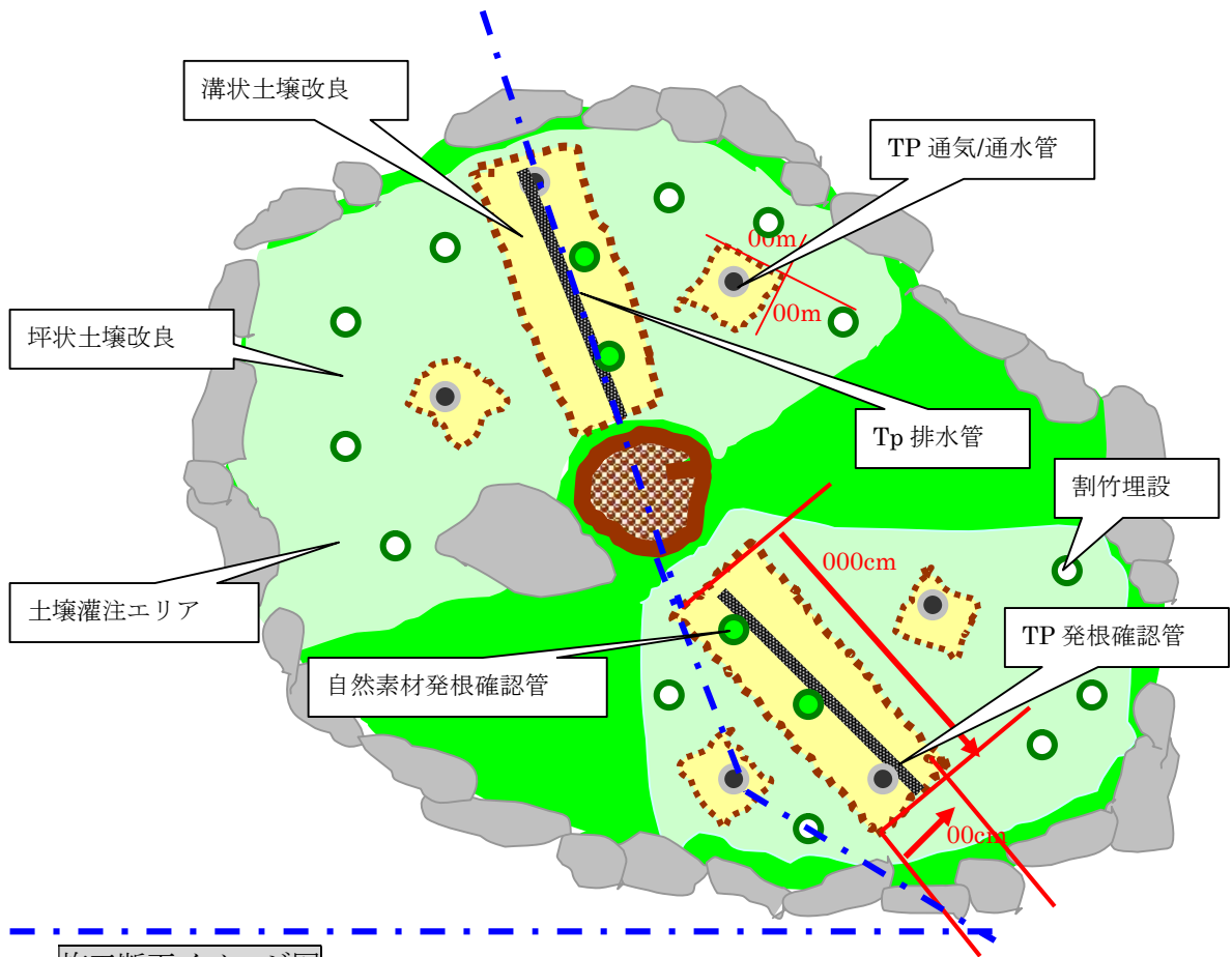
施工断面イメージ図
